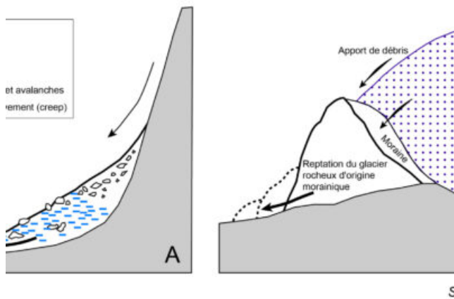
Fig. 1 – Modèles de développement de glaciers rocheux
