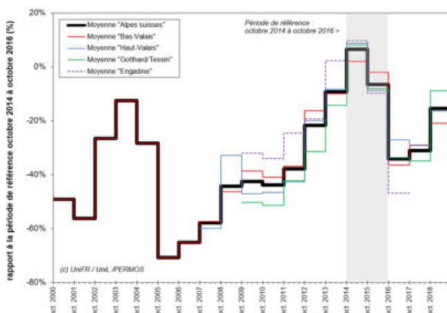
Fig. 4 – Vitesse horizontale de surface annuelle
