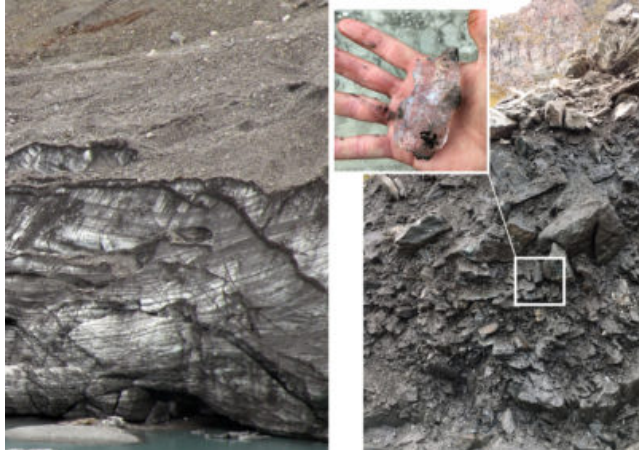
Fig. 9 – Glaciers rocheux et glaciers couverts
