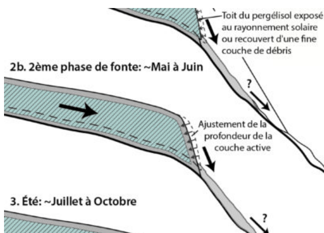
Fig. 7 – Front de glacier rocheux pendant différentes périodes d'activité
