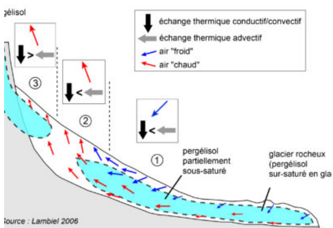
Fig. 3 – Circulation d'air ascendante dans un éboulis
