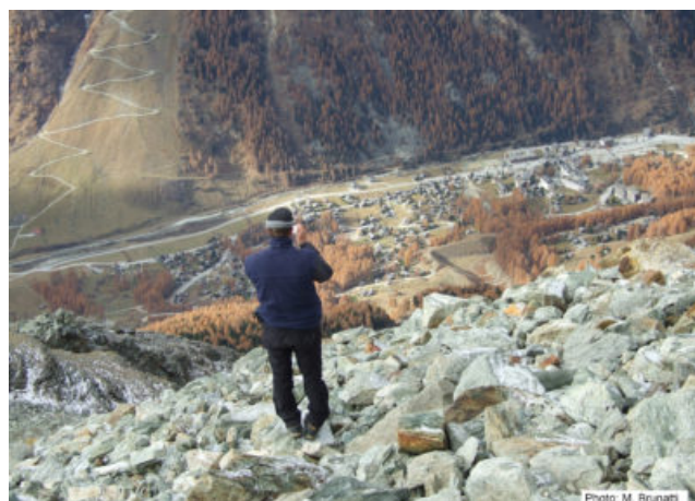
Fig. 3 – Glacier couvert du Bonnard (VS)
