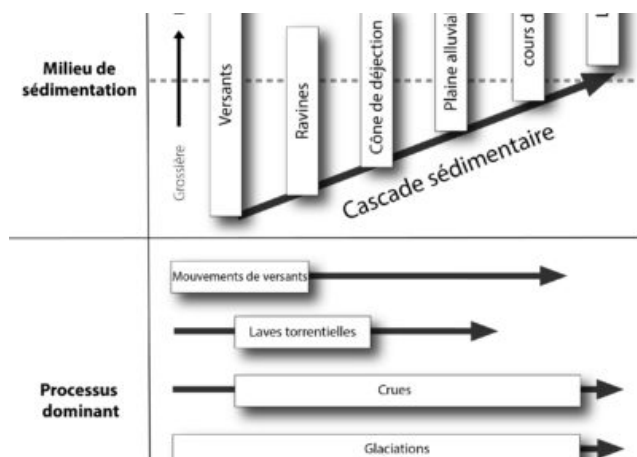
Fig. 2 – Milieux de sédimentation et les processus de transferts
