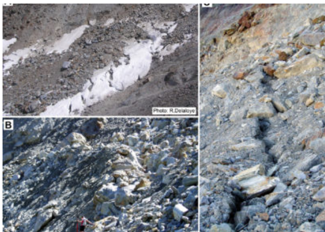
Fig. 2 – Déstabilisation d'un glacier rocheux
