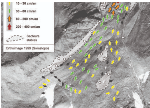
Fig. 1 – Vitesses de déplacement de blocs à la surface d'un glacier rocheux
