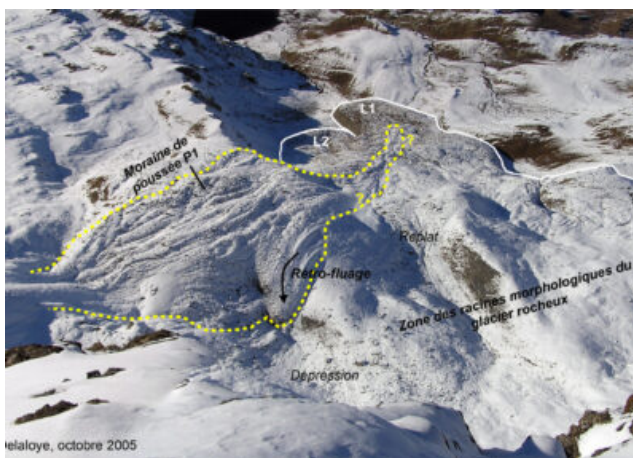
Fig. 2 – Glacier rocheux et moraine de poussée
