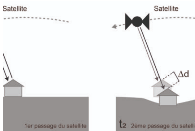
Fig. 5 – Interférométrie radar satellitaire différentielle
