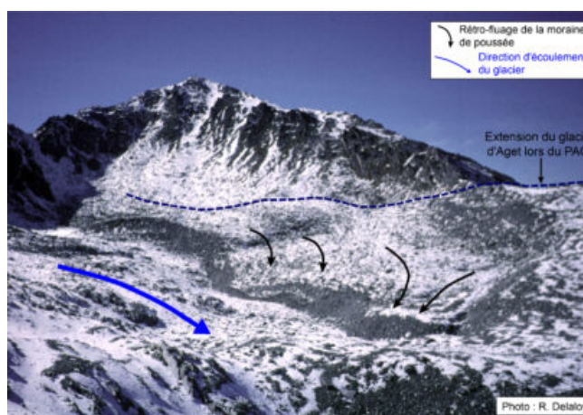
Fig. 5 – Rétro-fluage d'une moraine de poussée dans la marge proglaciaire
