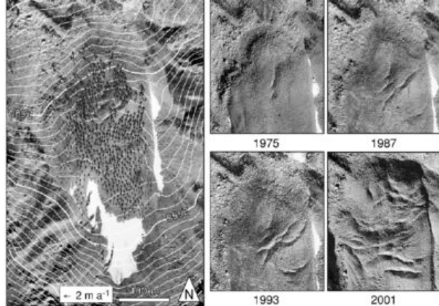
Fig. 3 – Instabilité de la tête d'un glacier rocheux
