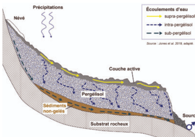
Fig. 4 – Fonctionnement hydrologique d'un glacier rocheux
