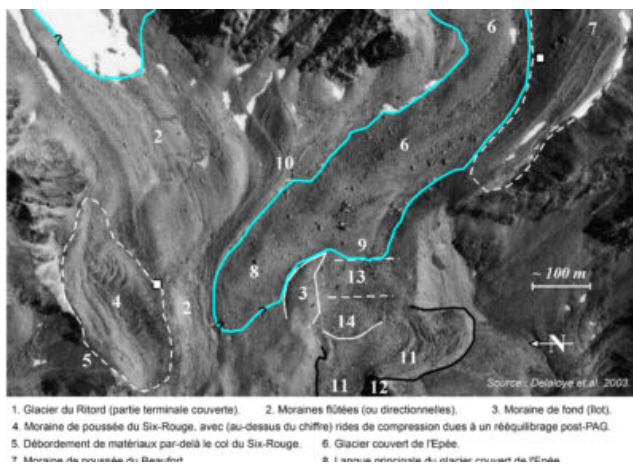
Fig. 1 – Aspects géomorphologiques d'une marge proglaciaire
