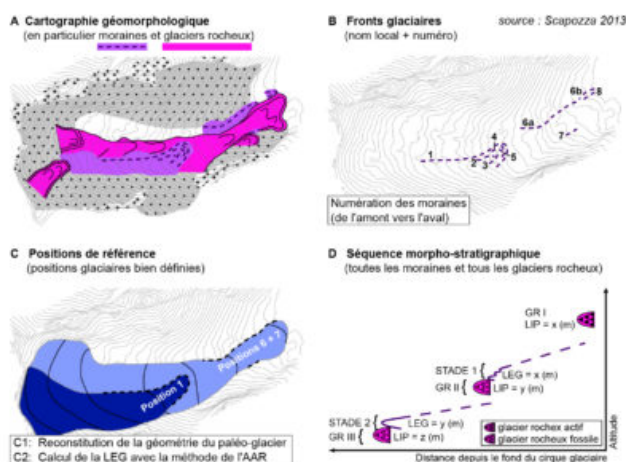
Fig. 2 – Datation relative des glaciers rocheux fossiles
