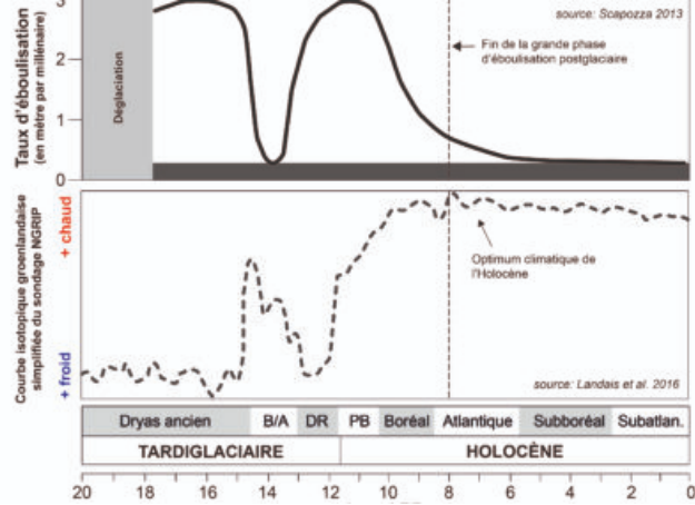
Fig. 6 – Evolution du taux d'ébouilisation et courbe isotopique groenlandaise
