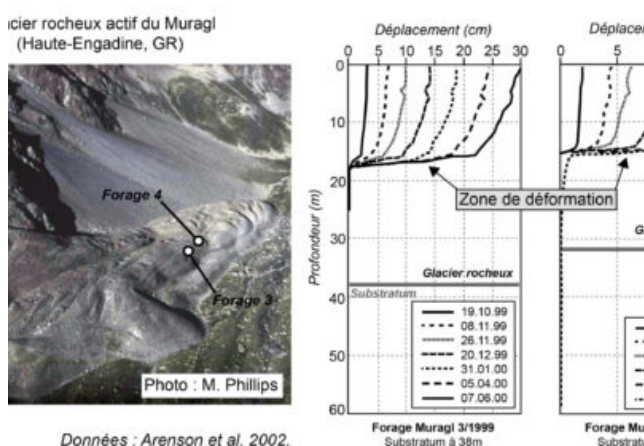
Fig. 2 – Déformation horizontale d'un glacier rocheux
