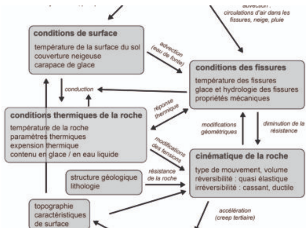
Fig. 2 – Interactions entre l’atmosphère et les parois rocheuses contenant du pergélisol
