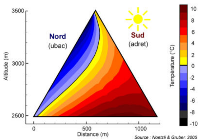
Fig. 3 – Champ thermique dans une montagne
