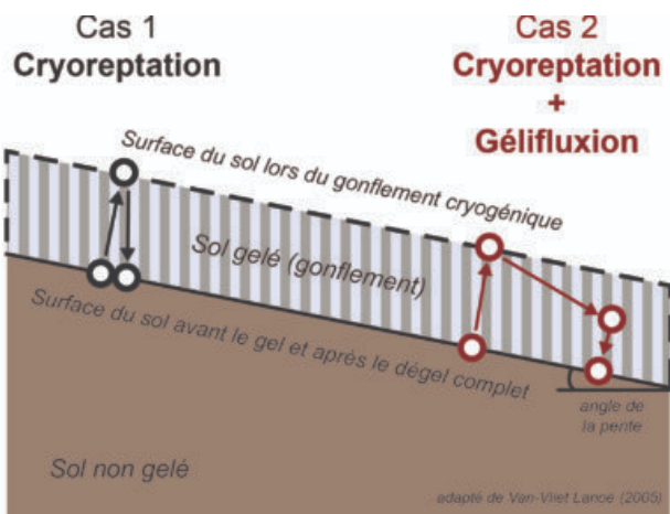
Fig. 1 – Trajectoire d’une particule lors de gel-dégel
