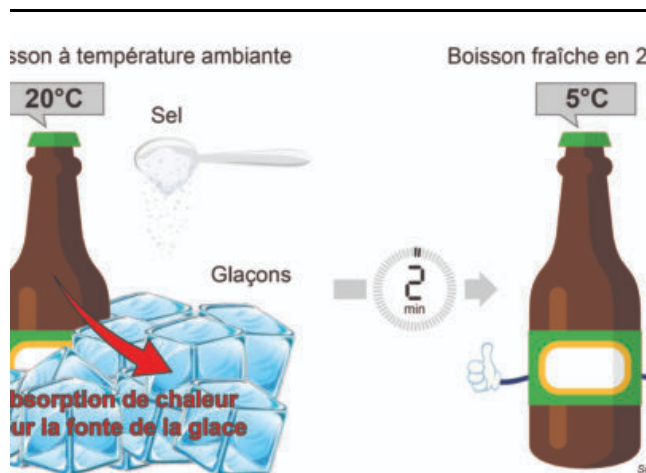
Fig. 1 – Principe de transfert de chaleur lors de la fonte de la glace
