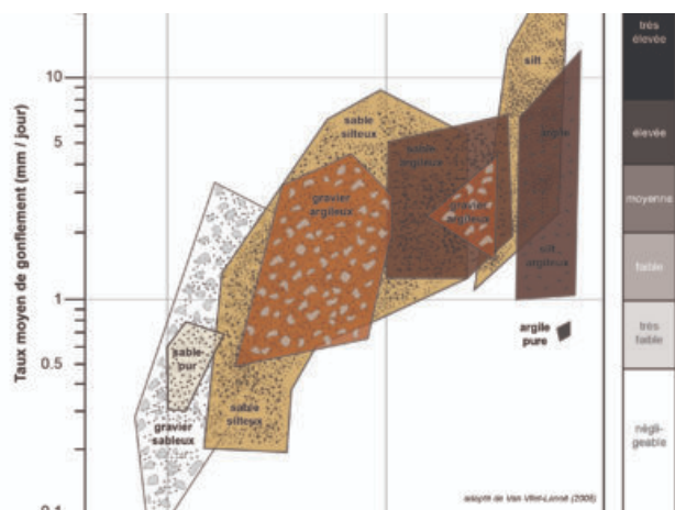
Fig. 2 – Gélivité et taux moyen de gonflement
