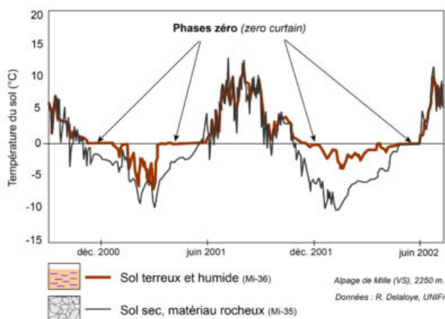
Fig. 2 – Phases de gel-dégel
