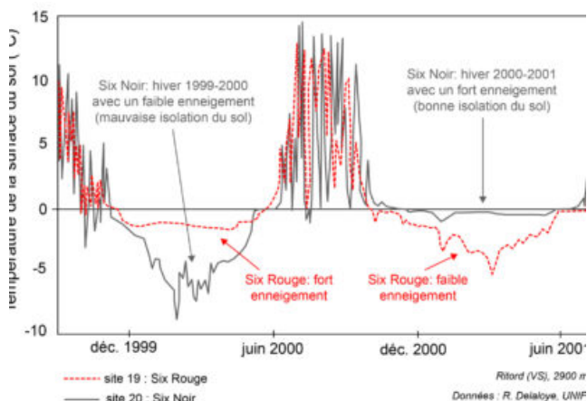
Fig. 3 – Variations des conditions thermiques
