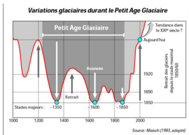
Fig. 1 – Fluctuations glaciaires pendant le Petit Age Glaciaire
