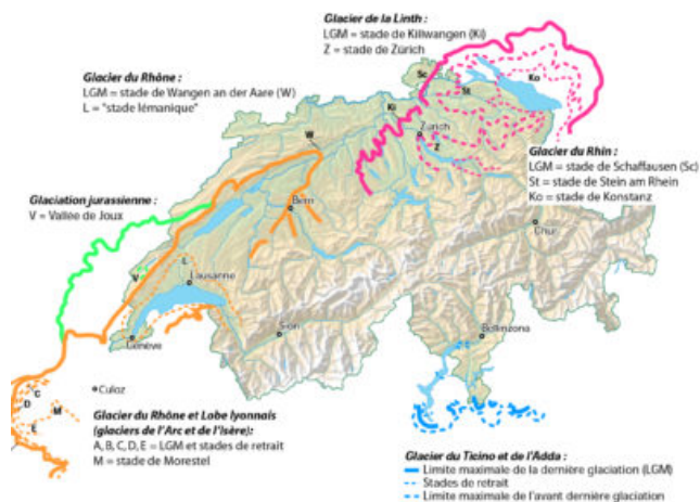
Fig. 3 – Dernier maximum glaciaire et principaux stades de retrait
