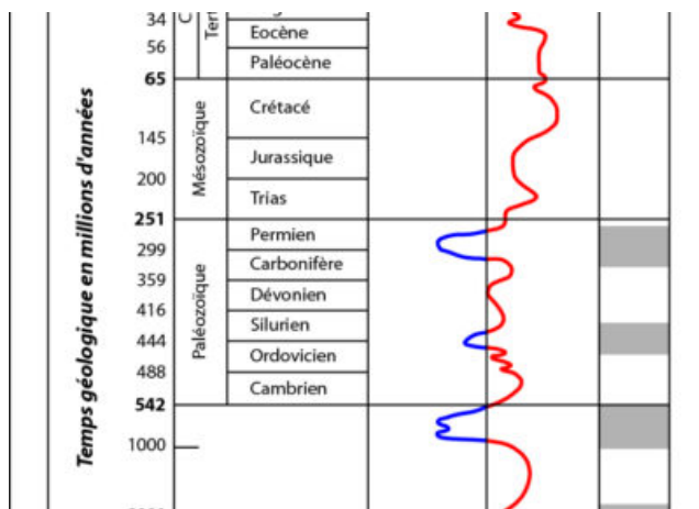
Fig. 1 – Evolution des températures pendant l’histoire de la Terre
