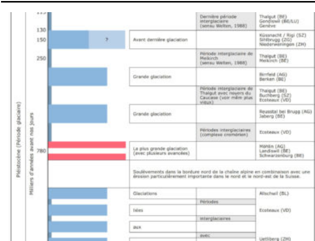
Fig. 1 – Chronologie des principales glaciations
