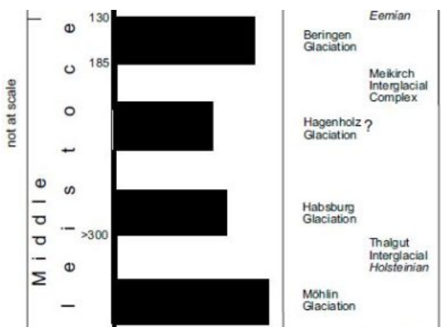
Fig. 2 – Histoire glaciaire de la Suisse
