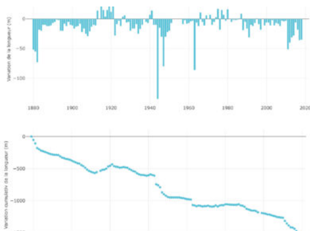
Fig. 2 – Longueur du glacier du Rhône (VS)
