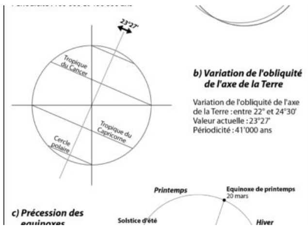
Fig. 1 – Cycles de Milankovitch
