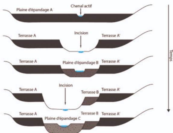
Fig. 6 – Formation de terrasses fluvio-glaciaires
