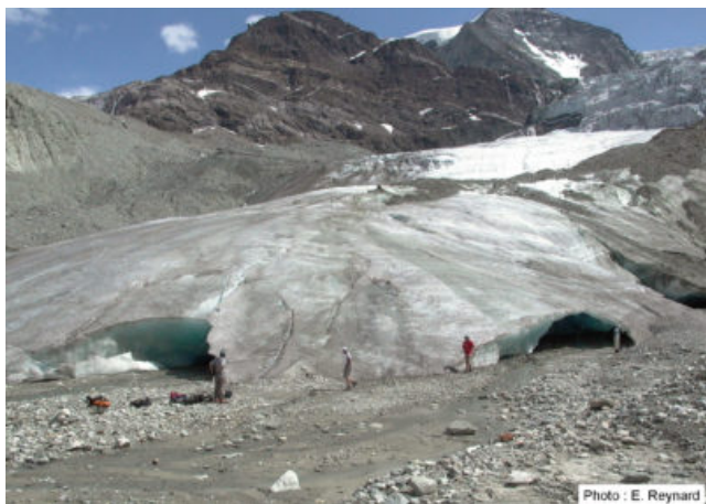
Fig. 1 – Partie frontale d'un glacier
