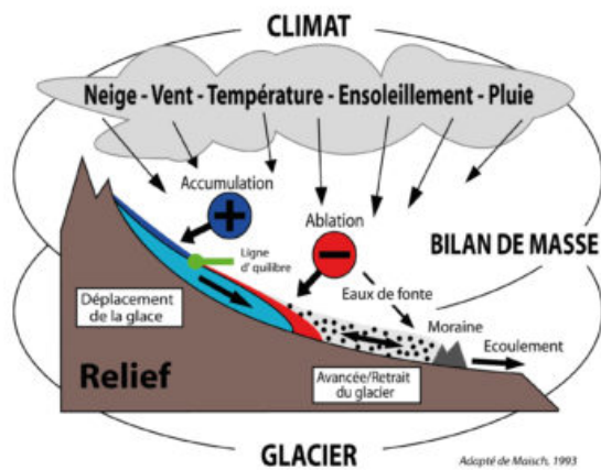
Fig. 1 – Glacier comme système hydroclimatique.
