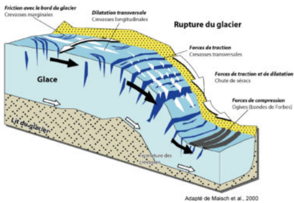
Fig. 1 – Types de crevasses dans un glacier alpin
