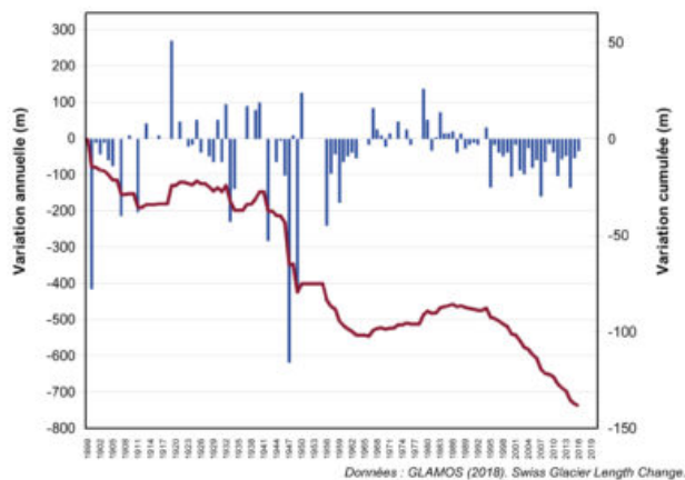
Fig. 4 – Longueur du glacier de Basòdino (TI)
