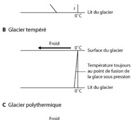
Fig. 1 – Profils de température
