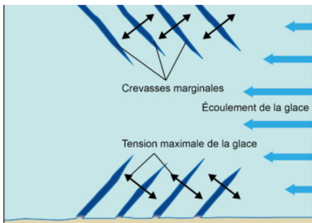
Fig. 2 – Formation des crevasses marginales
