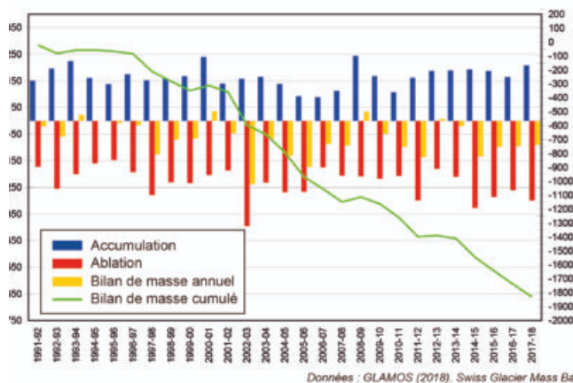
Fig. 2 – Bilan de masse d'un glacier
