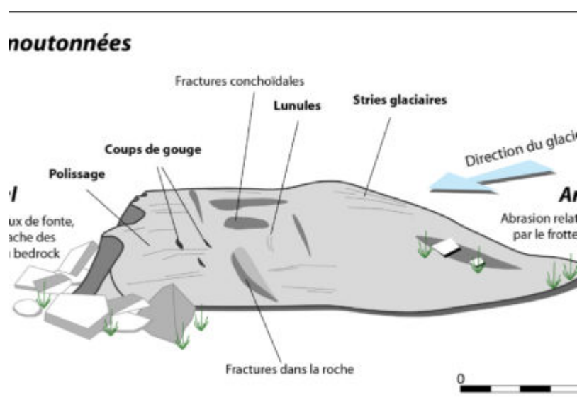
Fig. 1 – Dissymétrie des roches moutonnées liées à l'arrachement à l'aval de l'obstacle (adapté de Maisch et al., 1993).
