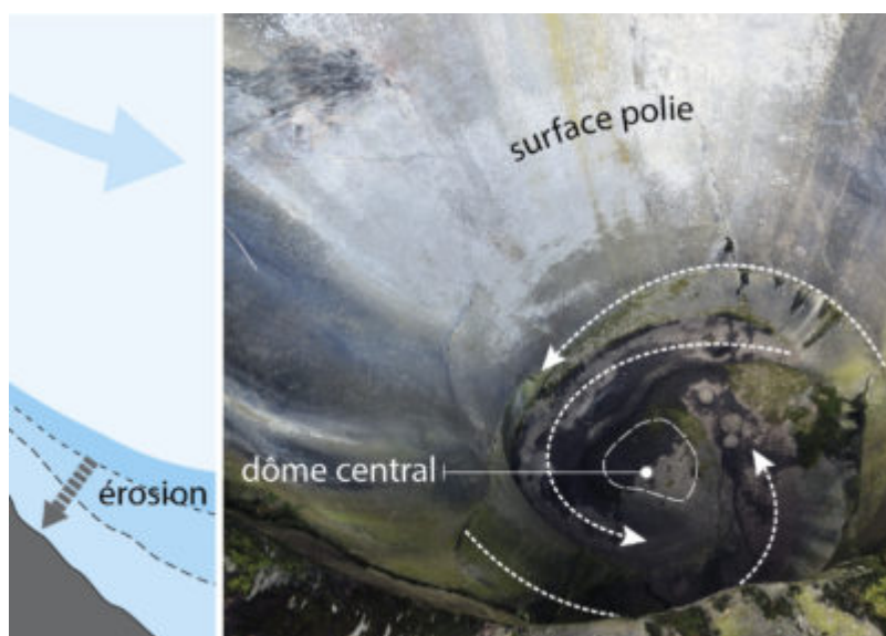
Fig. 7 – Les parois et le fond de la marmite gardent la trace de l'écoulement turbulent de l'eau descendant en spirale. Exemple : Marmite glacière des Caillettes , Bex (VD).
